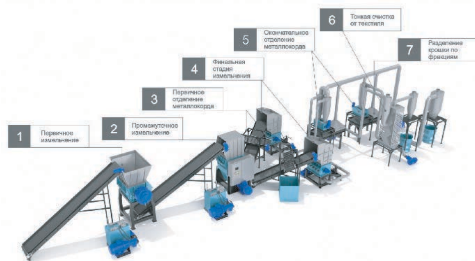
Линии по переработке шин
