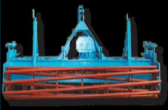
Культиватор фрезерный предназначен для предпосевной подготовки почвы с выравниванием и прикатыванием основной обработки, плугами и др. орудиями
